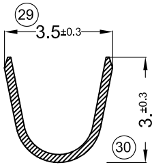
SECC. D-D
